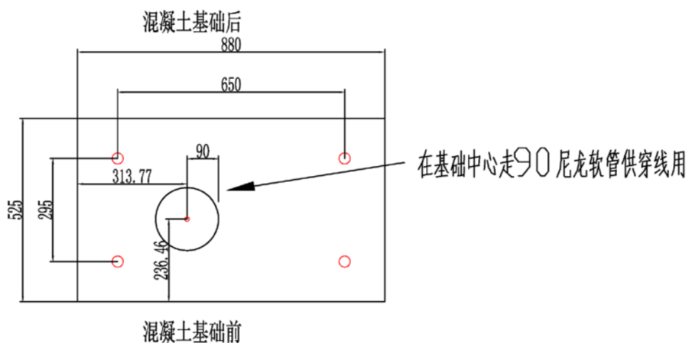
水泥基础尺寸
